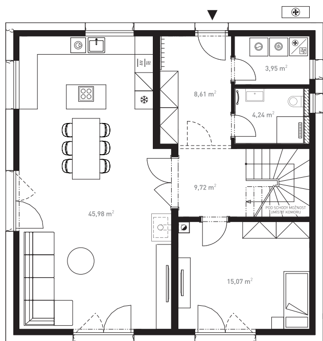
10,42 m Přízemí
